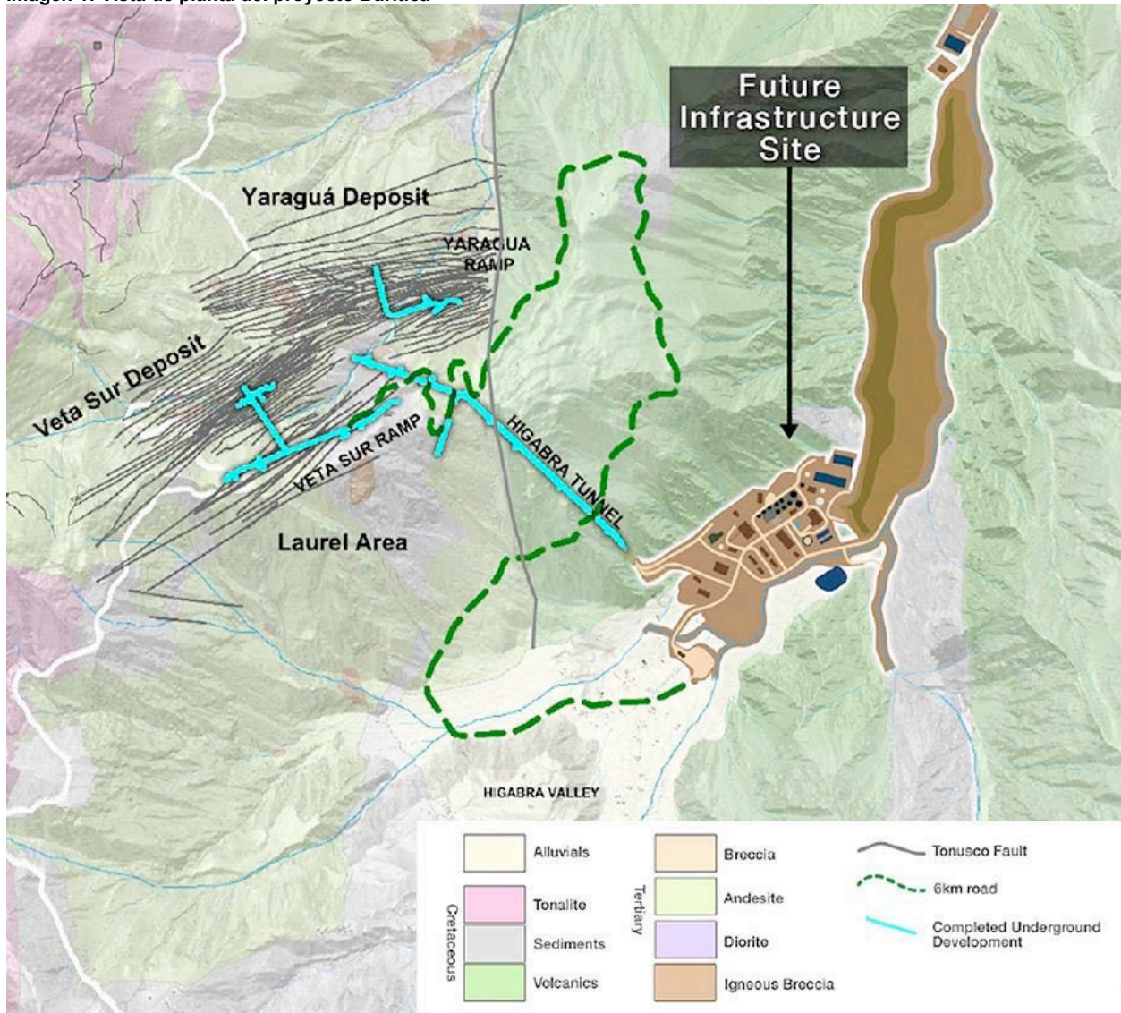
Imagen 1: Vista de planta del proyecto Buriticá
